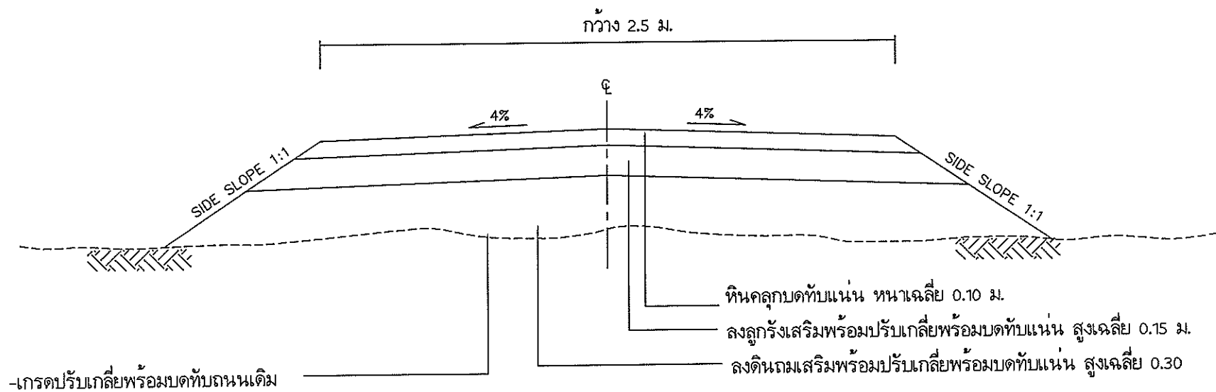
รูปตัดตามขวาง ถนนหินคลุก
